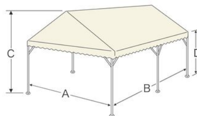
屋型テントフレーム
